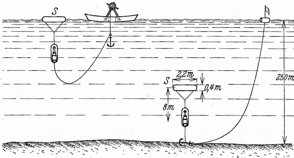
Fig. 6. Die „schwebende“ Verankerung des Apparates.
