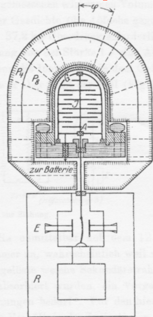
Fig. 1. Hochdruckionisationsgefäß J mit Drahtgitter G und Aufhänger A. Darum 12 cm Fe-Panzer ( P_4 , P_8 ), darunter Wulfsches Einfeldenelektrometer E mit Registriervorrichtung R.
