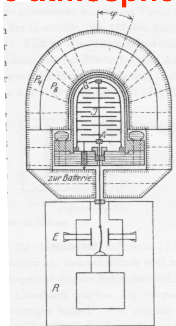
Fig. 1. Hochdruckionisationsgefäß J mit Drahtgitter G und Aufhänger A. Darum 12 cm Fe-Panzer ( P_4 , P_8 ), darunter Wulfsches Einfeldenelektrometer E mit Registriervorrichtung R.
