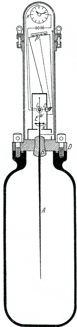
Fig. 1. Aufbau des wasserdichten Registrierapparates.
