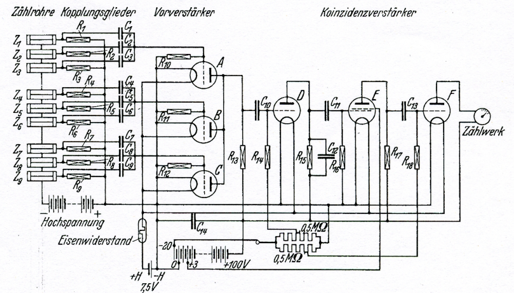
Fig. 2. Schaltschema des Koinzidenzverstärkers.
